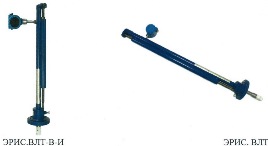
Рисунок 2 – Общий вид датчиков расхода ЭРИС модификации ВЛТ
