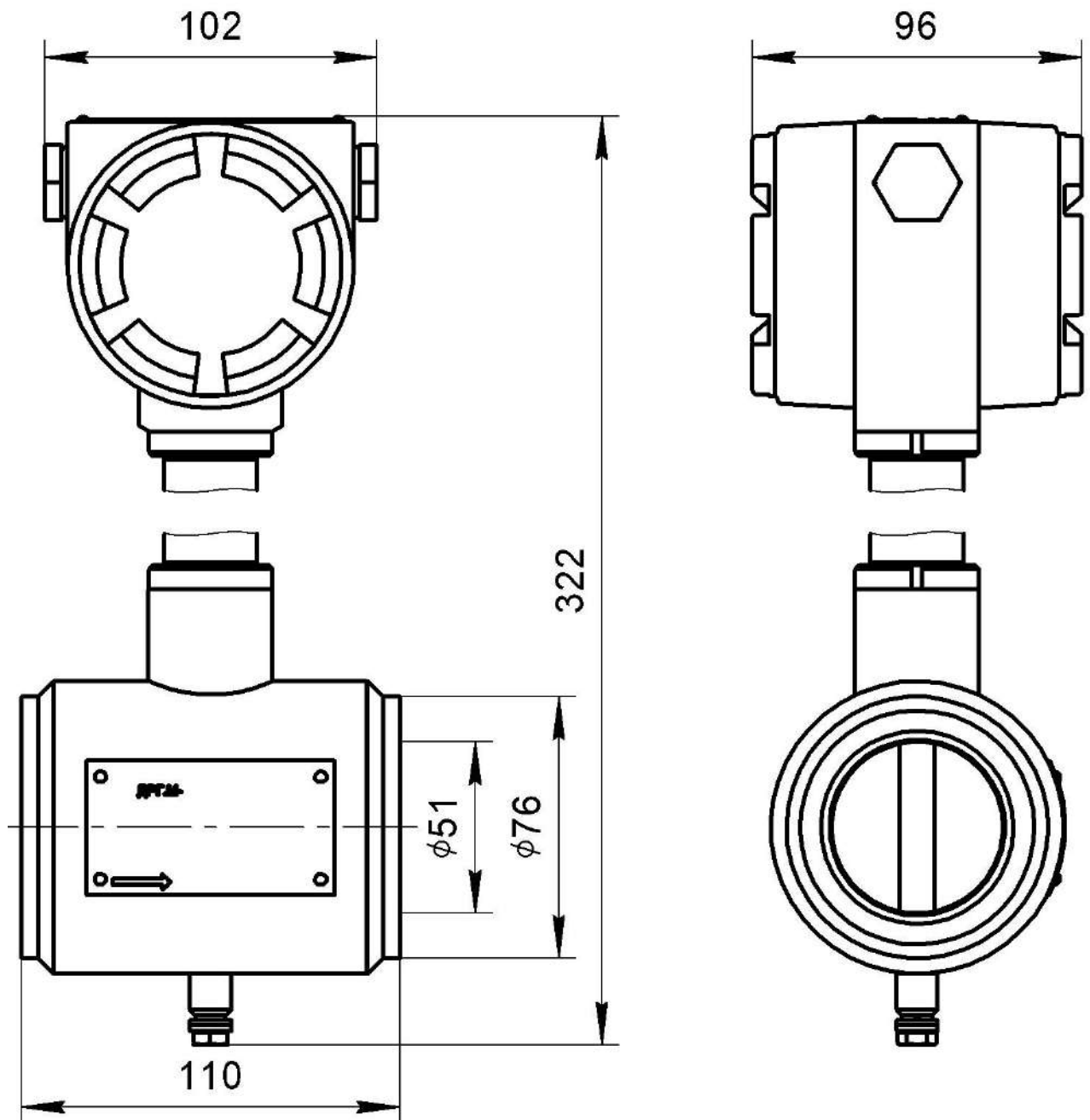
Рисунок А.7 – Датчик расхода ДРГ.М-800 с датчиком изгибающего момента пьезоэлектрическим. Общий вид
