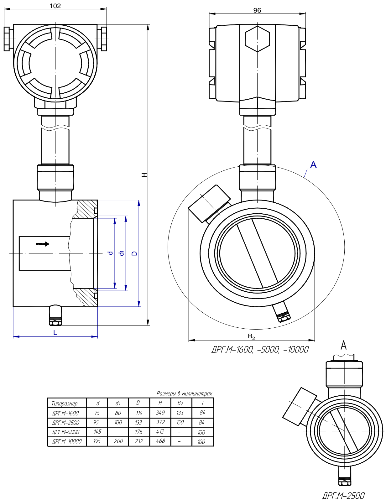
Рисунок А.3 – Датчик расхода DRG.M-1600, -2500, -5000, -10000 с датчиками давления пьезоэлектрическими. Общий вид
