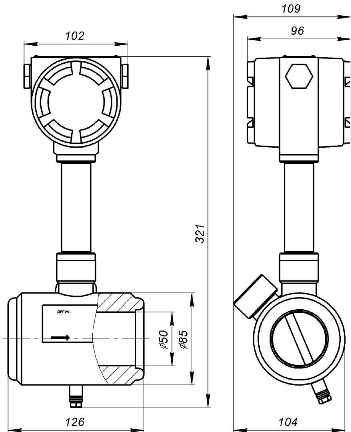
Рисунок А.5 – Датчик расхода ДРГ.М-800 на 20, 25 МПа с датчиками давления пьезоэлектрическими. Общий вид
