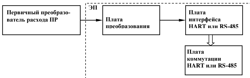
Рисунок 1б - Структурная схема датчика расхода с цифровым выходом
