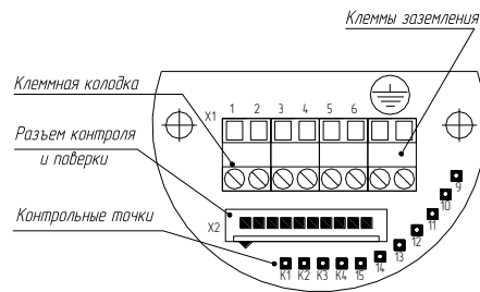
Рисунок 2 - Плата коммутации
