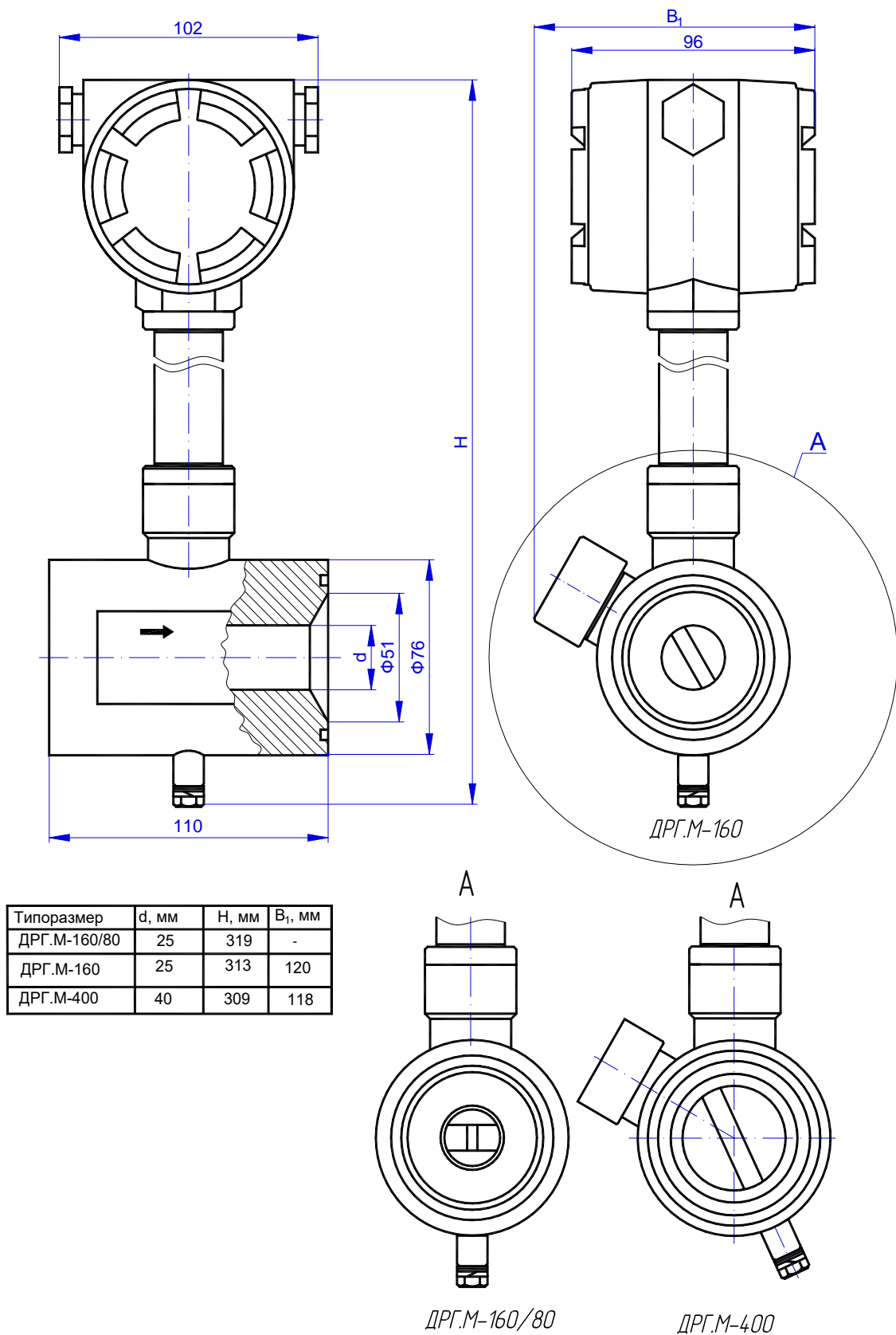
Рисунок А.1 – Датчик расхода газа ДРГ.М-160/80, -160, -400 с датчиками давления пьезоэлектрическими. Общий вид
