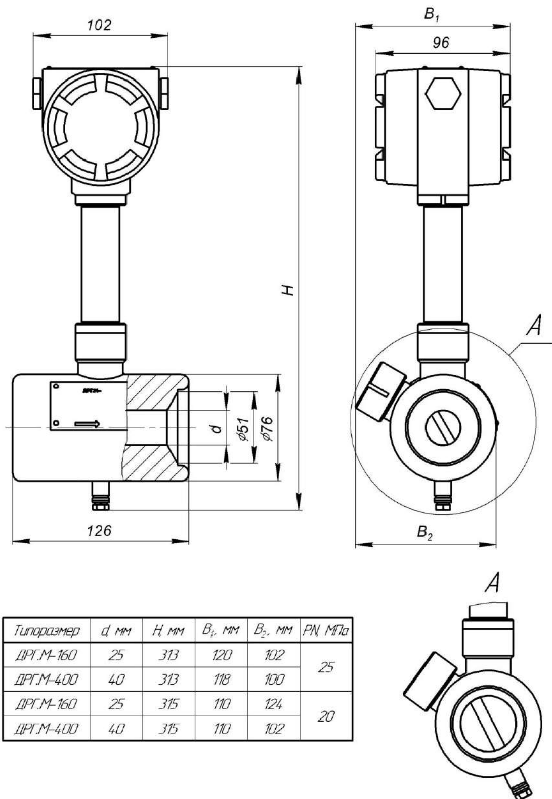
Рисунок А.4 – Датчик расхода ДРГ.М-160, -400 на 20, 25 МПа с датчиками давления пьезоэлектрическими. Общий вид
