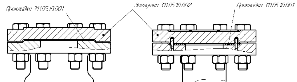
Установка заглушки
